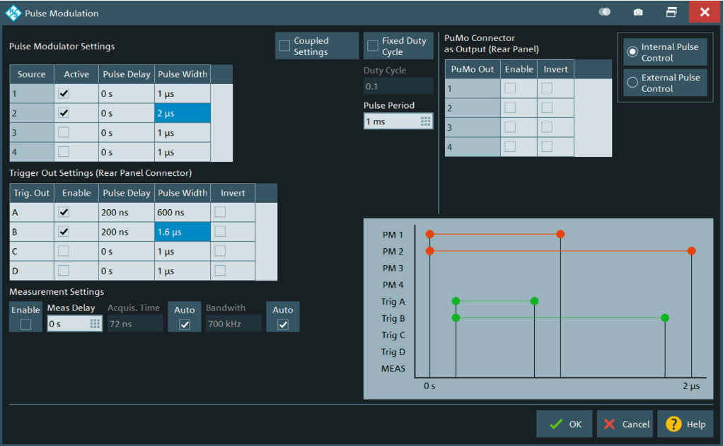
Конфигурация параметров для импульсных измерений
