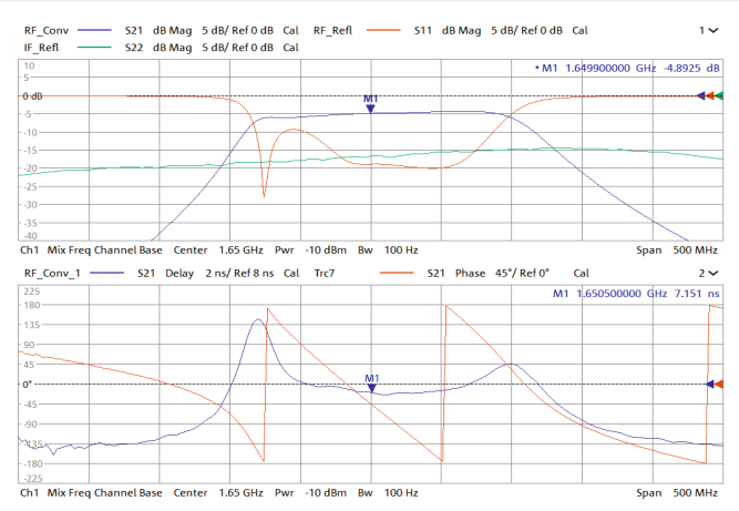
Результаты измерения параметров преобразователя, включая потери на отражение, потери на преобразование, фазу и ГВЗ
